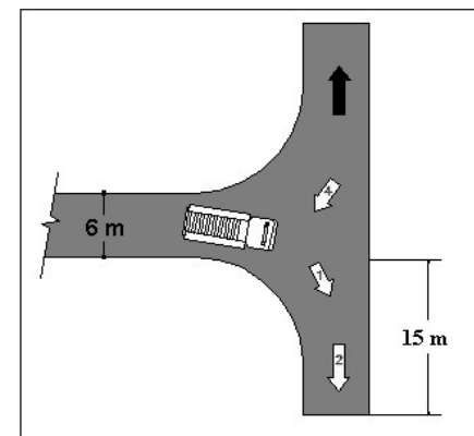
Figura 4 – Retorno em T
