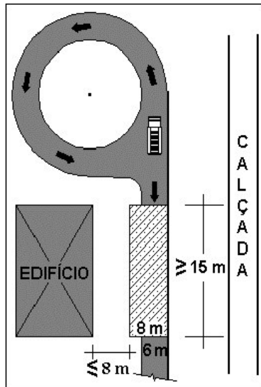
Figura 7 – Faixa de estacionamento
